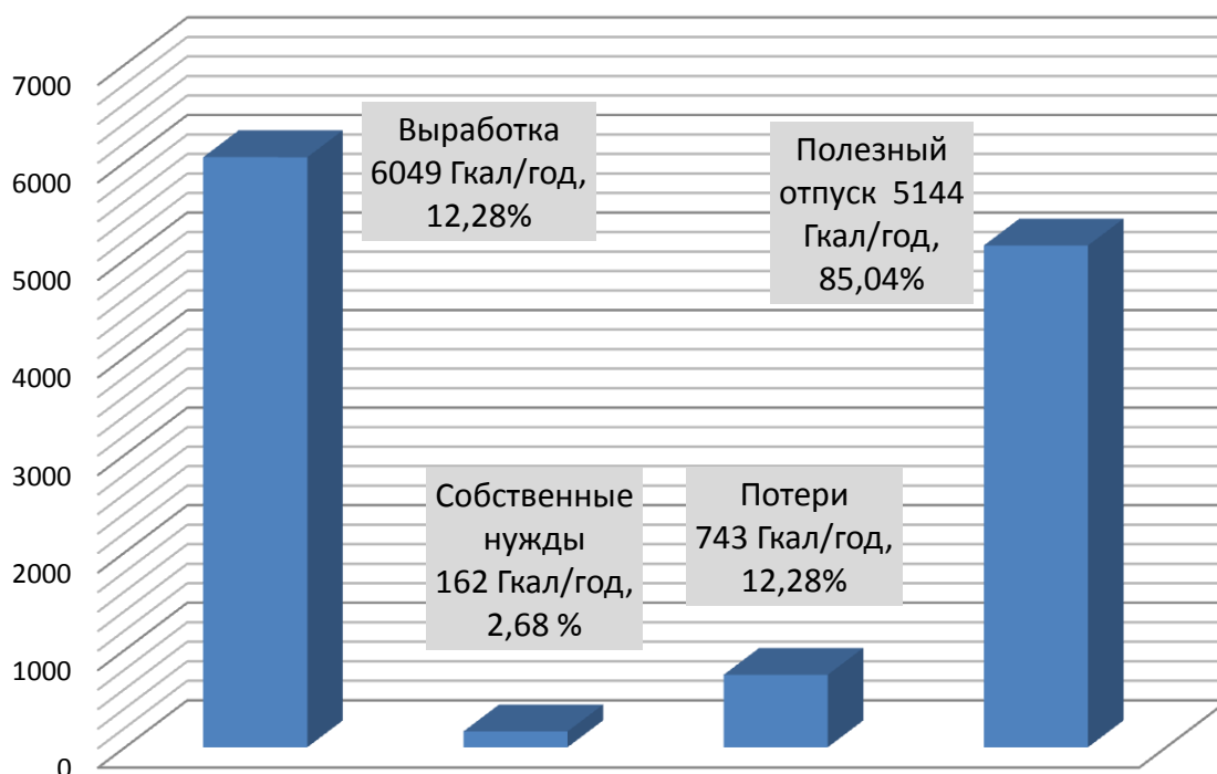
Рис. 1. Информация о тепловом балансе котельной с. Козиха.
